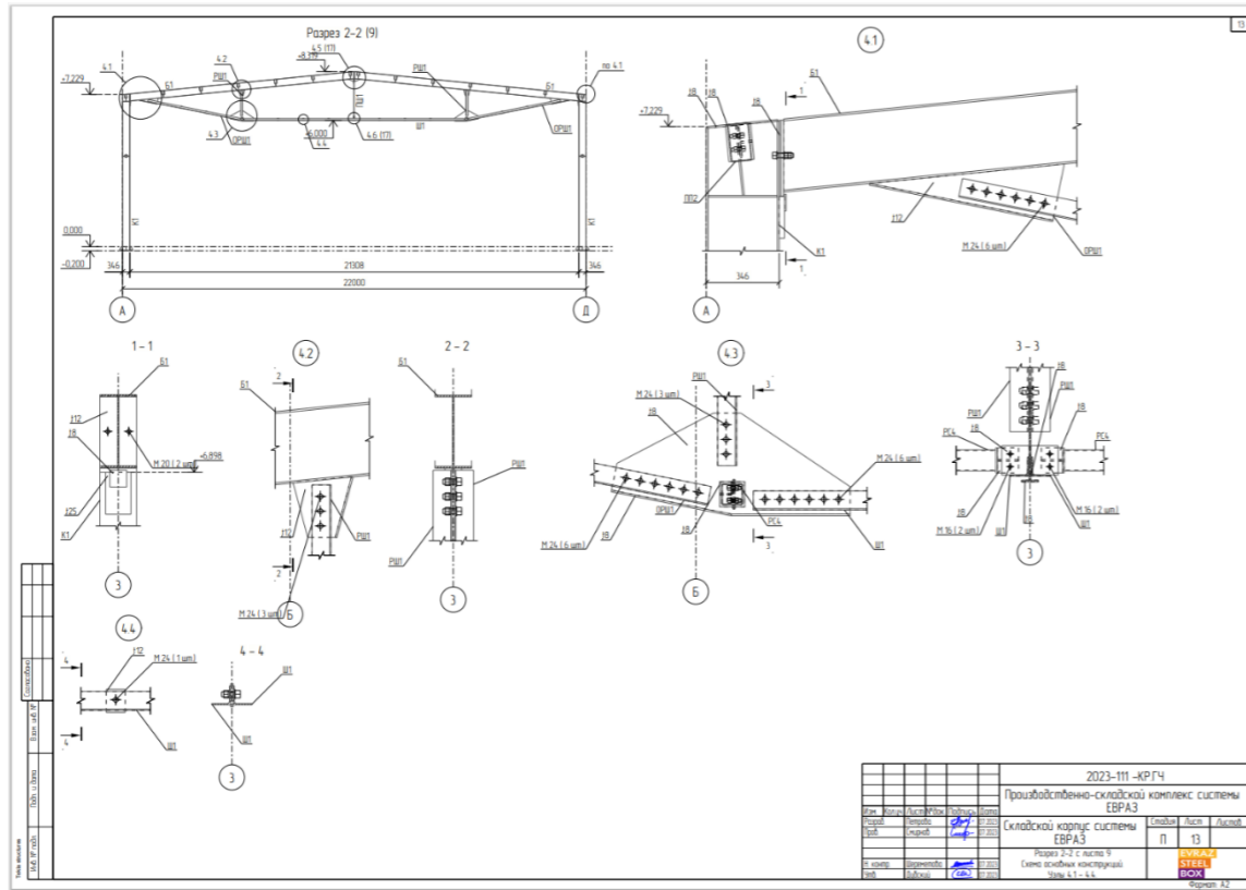
РАЗРЕЗ 2-2
